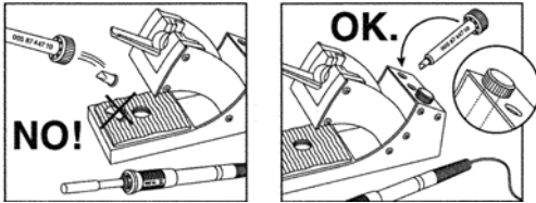
Der Lötspitzenwechsel am Lötencil WSP 80
